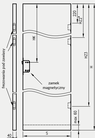
Skrzydła bezprzylgowe rozwierne Standard 10, Modern, Plus
