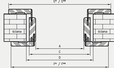
Przekrój poprzeczny TUN
