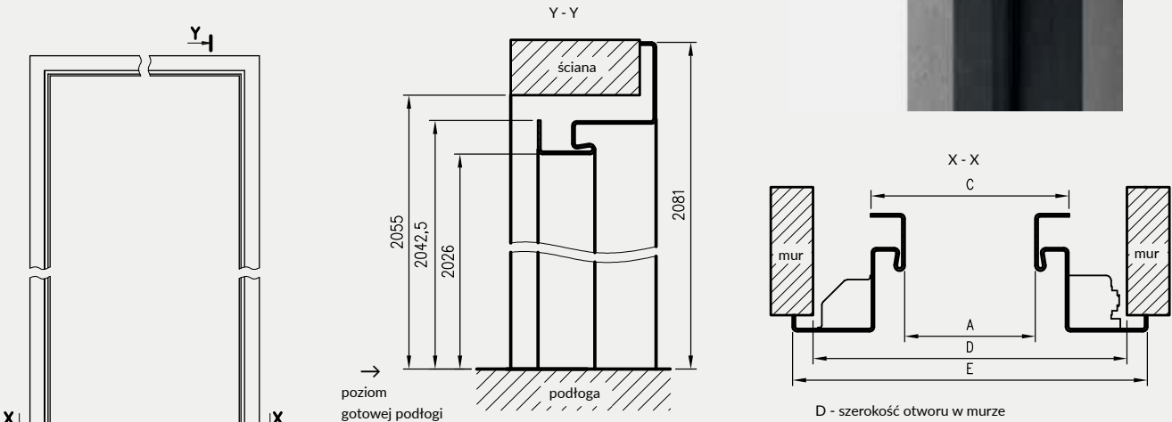
wymiary dla drzwi jednoskrzydłowych
