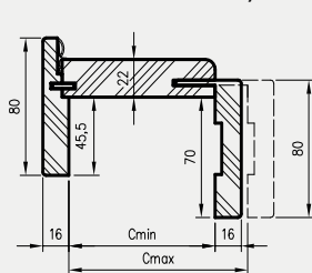
Profil ościeżnicy
