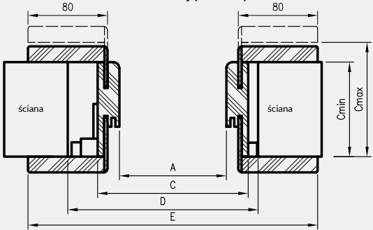
B-B Przekrój poziomy
