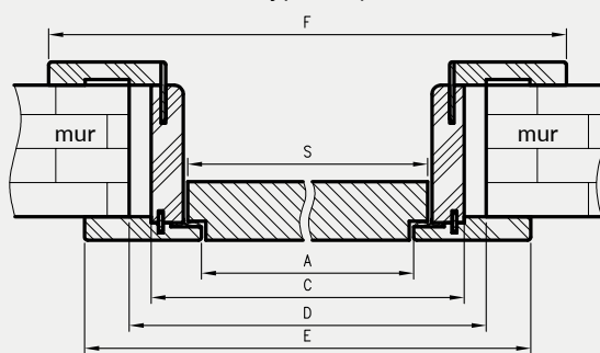
Przekrój poziomy ORO
