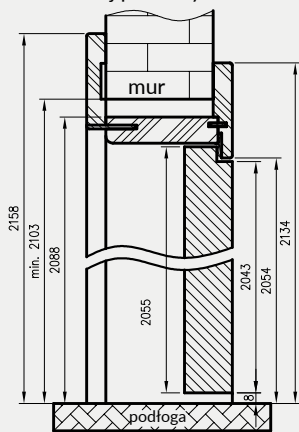
Przekrój pionowy ORO
