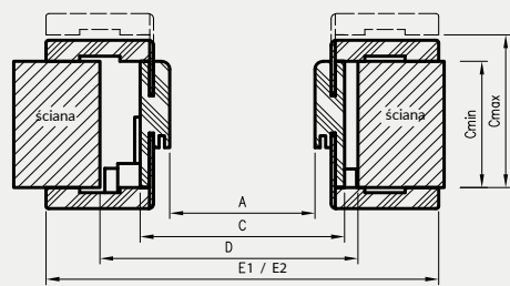
Przekrój poziomy ORB
