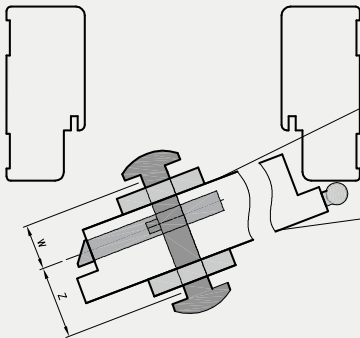
Rys. Dobór wymiaru wkładki z gałką
