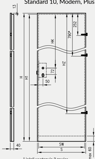
Skrzydła bezprzylgowe rozwierne Standard 10, Modern, Plus
