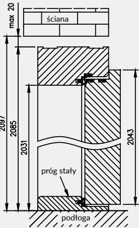
Ościeznica drewniana do drzwi Athos z progiem stałym
