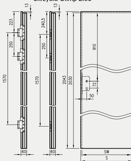
Skrzydła Olimp EI60**
