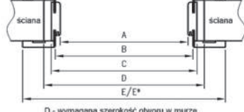
Przekrój poziomy OR
