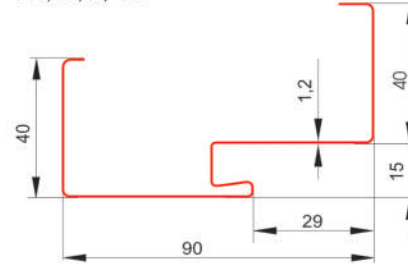
Ościeznica asymetryczna FD/21/C/40
