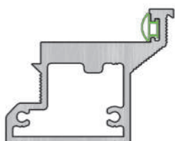
OŚCIEŻNICA ALUMINIOWA PRZYLGOWA OTWIERANA DO WEWNĄTRZ
