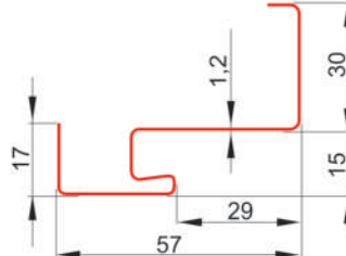
Ościeznica narożna FD/25/21/N/O
