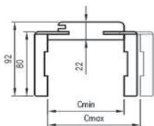
Przekrój OR z kątem T80
