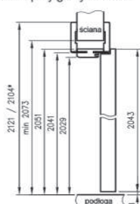
Przekrój pionowy drzwi przylgowych z OR
