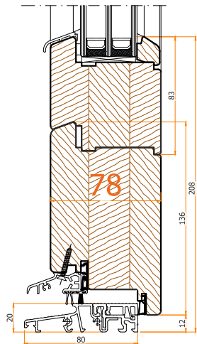
PROFIL 78 - THERMOLINE
