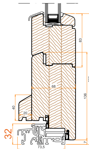
Próg aluminiowy GUTMANN 74/32 TI
