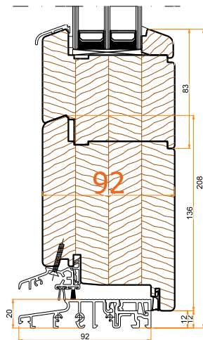
PROFIL 92 - ECOTHERM
