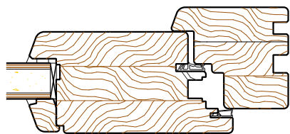
Profil Softline
