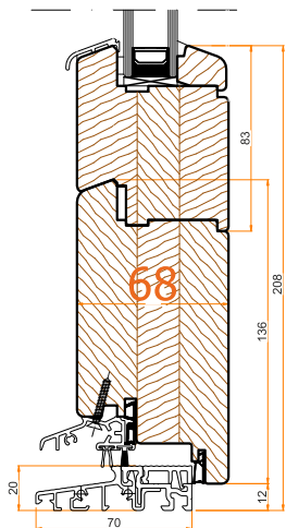
PROFIL 68 - ECOLINE
