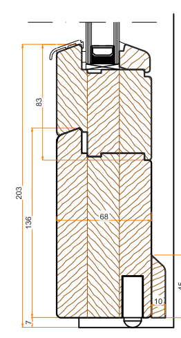
Uszczelka progowa DEVENTER DSD 1530
