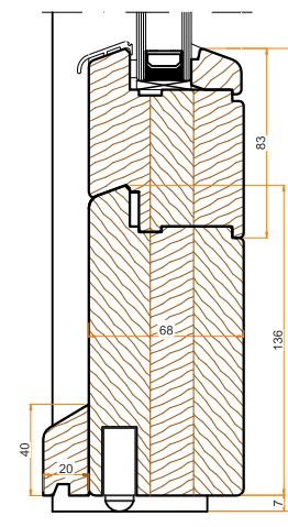
Uszczelka progowa DEVENTER DSD 1530
