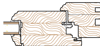
Profil Retro
