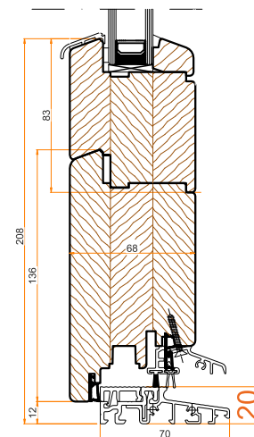
Próg aluminiowy TS 57022
